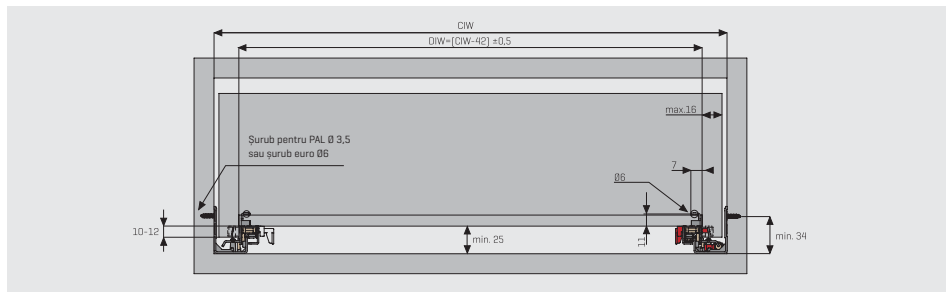
Amplasarea șuruburilor pentru glistiere Fixare cu pin
