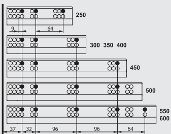
Amplasarea șuruburilor pentru glistiere Fixare cu conector
